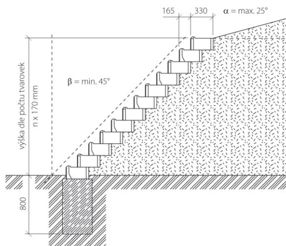
opěrná zeď, maximální možný sklon svahu 45^\circ
