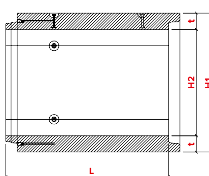
PODÉLNÝ ŘEZ
