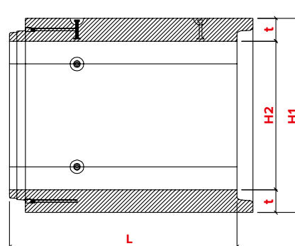
PODÉLNÝ ŘEZ
