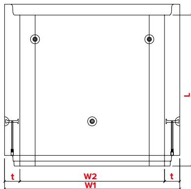
PŮDORYS
