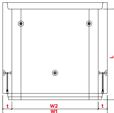
PŮDORYS
