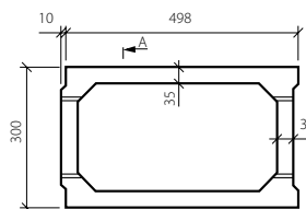
BEST ZTRACENÉ BEDNĚNÍ 30 – půdorys
