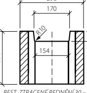
BEST ZTRACENÉ BEDNĚNÍ 30 – řez A-A
