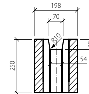
BEST ZTRACENÉ BEDNĚNÍ 20 – řez A-A
