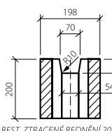
BEST ZTRACENÉ BEDNĚNÍ 20 – řez A-A
