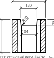
BEST ZTRACENÉ BEDNĚNÍ 25 – řez A-A
