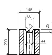
BEST ZTRACENÉ BEDNĚNÍ 15 – řez A-A
