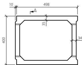
BEST ZTRACENÉ BEDNĚNÍ 40 – půdorys
