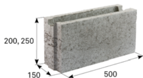
BEST ZTRACENÉ BEDNĚNÍ 15
