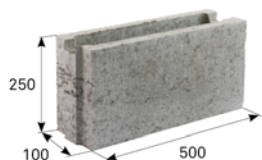
BEST ZTRACENÉ BEDNĚNÍ 10
