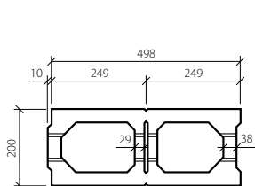
BEST ZTRACENÉ BEDNĚNÍ 20 - připraveno na dělení
