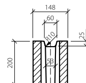
BEST ZTRACENÉ BEDNĚNÍ 15 - řez A-A
