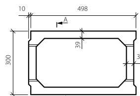
BEST ZTRACENÉ BEDNĚNÍ 30 - půdorys
