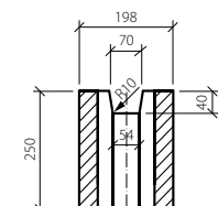
BEST ZTRACENÉ BEDNĚNÍ 20 - řez A-A
