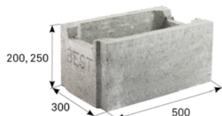
BEST ZTRACENÉ BEDNĚNÍ 30
