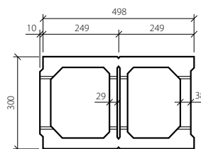
BEST ZTRACENÉ BEDNĚNÍ 30 - připraveno na dělení
