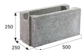
BEST ZTRACENÉ BEDNĚNÍ 25
