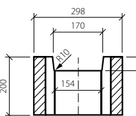
BEST ZTRACENÉ BEDNĚNÍ 30 - řez A-A
