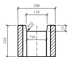
BEST ZTRACENÉ BEDNĚNÍ 30 – řez A-A
