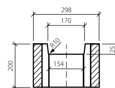
BEST ZTRACENÉ BEDNĚNÍ 30 – řez A-A
