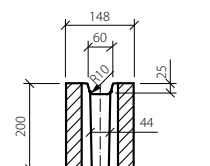
BEST ZTRACENÉ BEDNĚNÍ 15 – řez A-A
