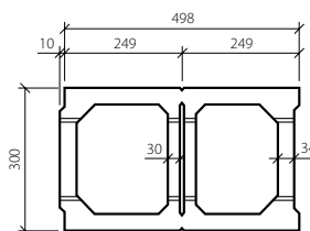
BEST ZTRACENÉ BEDNĚNÍ 30 – připraveno na dělení
