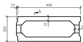
BEST ZTRACENÉ BEDNĚNÍ 20 – půdorys
