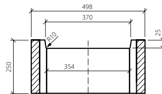
BEST ZTRACENÉ BEDNĚNÍ 50 – řez A-A
