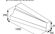
BEST ZASTÁVKOVÝ OBRUBNÍK přechodový 290/250
