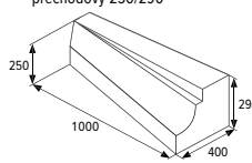
BEST ZASTÁVKOVÝ OBRUBNÍK přechodový 250/290
