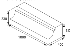
BEST ZASTÁVKOVÝ OBRUBNÍK náběhový 330/310
