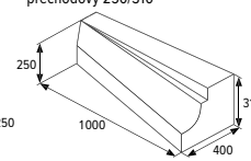
BEST ZASTÁVKOVÝ OBRUBNÍK přechodový 250/310
