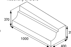
BEST ZASTÁVKOVÝ OBRUBNÍK náběhový 370/310
