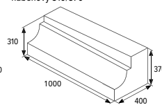
BEST ZASTÁVKOVÝ OBRUBNÍK náběhový 310/370
