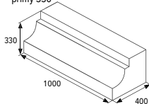
BEST ZASTÁVKOVÝ OBRUBNÍK přímý 330
