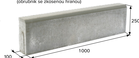
BEST SINIA III (obrubník se zkosenou hranou)
