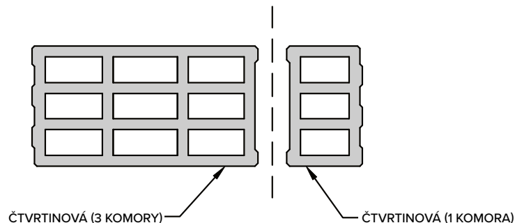
Tvarovky pro založení převazby rohu lze získat rozříznutím rohového bloku v místě svislé fazety.
