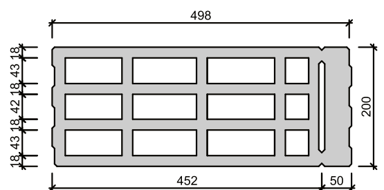
Broušená betonová tvárnice BR 20 Rohová 200×249×498 mm
