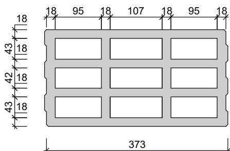
Broušená betonová tvárnice BR 20375 Základní 200×249×373 mm
