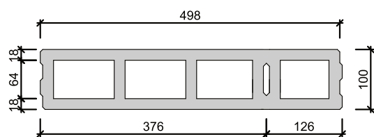
Broušená betonová tvárnice BR 10 Čtvrtinová 100×249×498 mm
