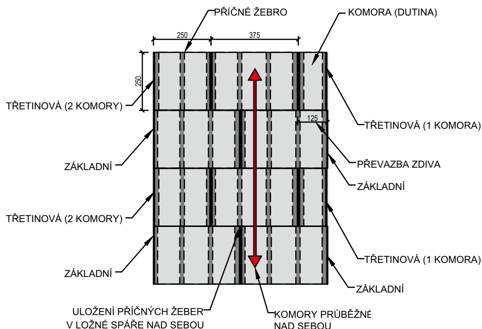
Broušené betonové tvárnice BR 25
