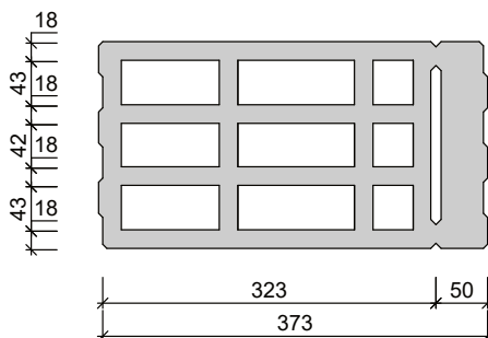
Broušená betonová tvárnice BR 20375 Rohová 200×249×373 mm
