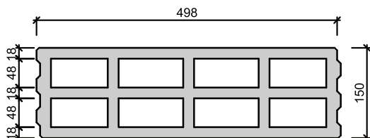
Broušená betonová tvárnice BR 15 Základní 150×249×498 mm
