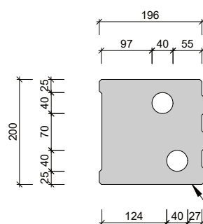
Broušená akustická betonová tvárnice BR 20 AKU
