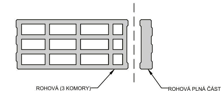
Tvarovky pro založení převazby rohu lze získat rozříznutím rohového bloku v místě svislé fazety.
