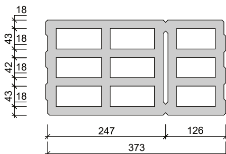
Broušená betonová tvárnice BR 20375 Třetinová 200×249×373 mm
