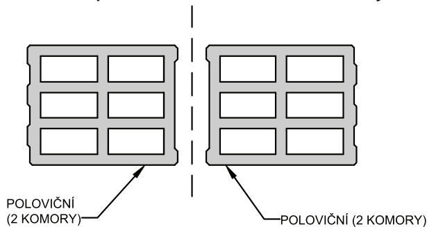
Tvarovky pro založení převazby ostění lze získat rozříznutím polovičního bloku v místě svislé fazety.
