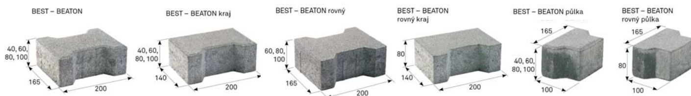
Skladebné rozměry
