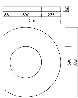
vyrovnávací prstenec TBV-Q 390/60
