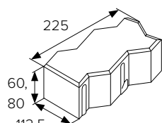
BEST BASE kraj
