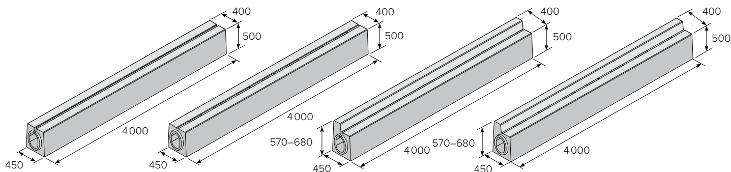
TROUBA S PRŮBĚŽNÝM ŠTĚRBINOVÝM ŽLABEM A OBRUBNÍKEM
