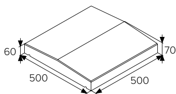
BEST ZÁKRYTOVÁ DESKA V sloupková (na sloupek 40x40 cm)
