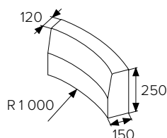
BEST MONO II R1 vnitřní
