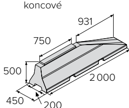
SVODIDLO MALÉ 50 koncové
