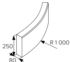
BEST LINEA R1 vnější
