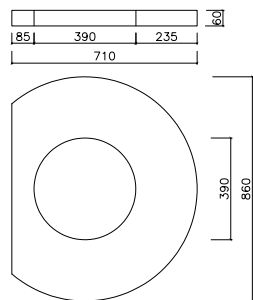
vyrovnávací prstenec TBV-Q 390/60
