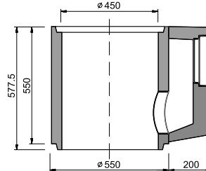
TBV-Q S/450/550 skruž se zápachovou uzávěrou DN 200 PVC
