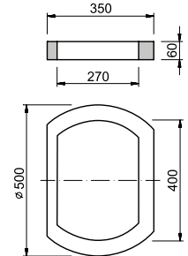
TBV-Q 10b/500×350/400×270/60 prstenec
