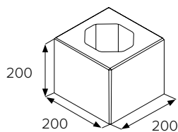
BEST MURO II
