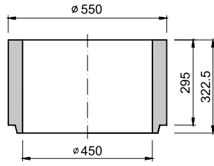
TBV-Q 5b/450/295 skruž horní
