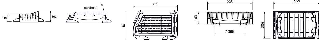
mříž + rám KM11RD pro přímé zabudování do Curb Kingu
