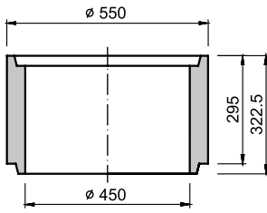
TBV-Q 3d/450/450 skruž s výtokem DN 200 bez vložky
