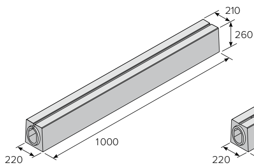
TROUBA S PRŮBĚŽNÝM ŠTĚRBINOVÝM ŽLABEM
