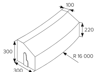
BEST RONDA R16 vnější
