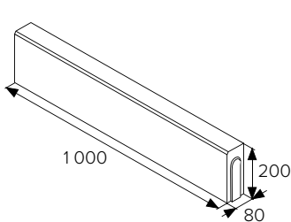
BEST LINEA III
