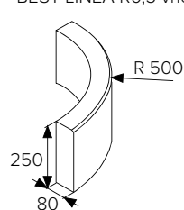
BEST LINEA R0,5 vnější
