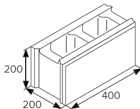
BEST LUNETA II (průběžný prvek)
