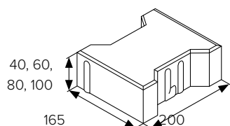
BEST BEATON rovný
