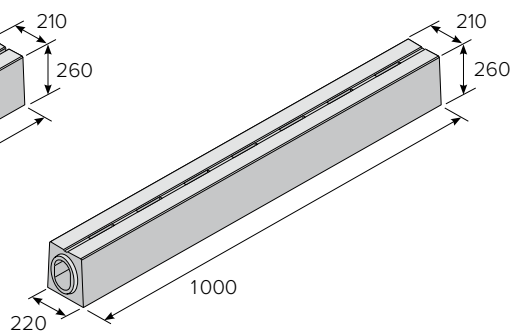
TROUBA S PŘERUŠOVANÝM ŠTĚRBINOVÝM ŽLABEM
