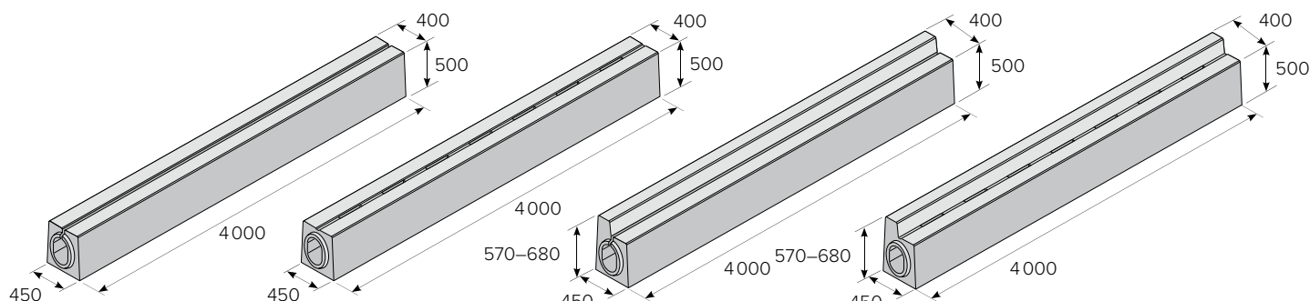
TROUBA S PRŮBĚŽNÝM ŠTĚRBINOVÝM ŽLABEM A OBRUBNÍKEM
