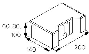
BEST BEATON rovný kraj
