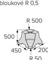
SVODIDLO MALÉ 50 obloukové R 0,5
