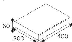
BEST ZÁKRYTOVÁ DESKA II průběžná
