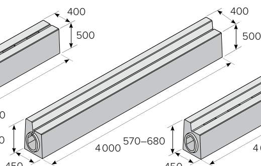
TROUBA S PRŮBĚŽNÝM ŠTĚRBINOVÝM ŽLABEM A OBRUBNÍKEM
