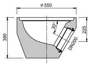
TBV-Q 1d/450/380 dno s vložkou DN 200 PVC
