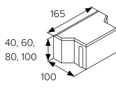
BEST BEATON rovný půlka
