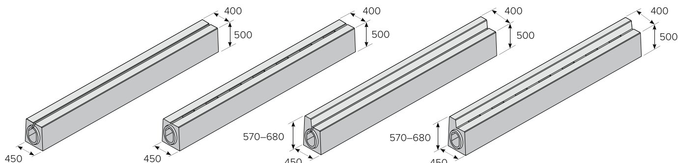
TROUBA S PRŮBĚŽNÝM ŠTĚRBINOVÝM ŽLABEM A OBRUBNÍKEM
