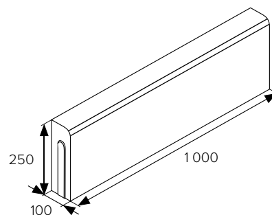
BEST SINIA III
