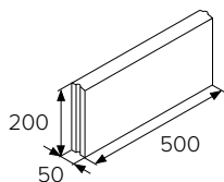
BEST PARKAN III
