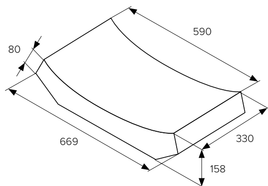
BEST ŽLAB I
