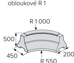
SVODIDLO MALÉ 50 obloukové R 1
