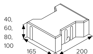
BEST BEATON rovný
