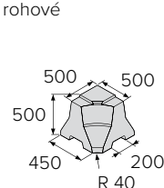
SVODIDLO MALÉ 50 rohové
