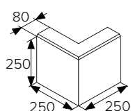
BEST LINEA rohová 90 vnější
