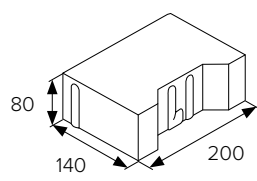
BEST BEATON rovný kraj
