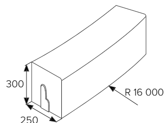
BEST KERBO R16 vnější
