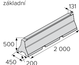
SVODIDLO MALÉ 50 základní
