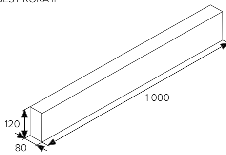
BEST ROKA II
