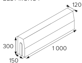
BEST MONO I
