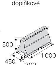
SVODIDLO MALÉ 50 doplňkové
