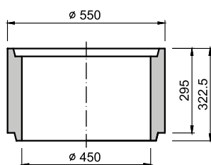
TBV-Q 6a/450/295 skruž středová
