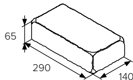
BEST KASKADA II
