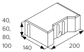
BEST BEATON rovný kraj
