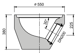
TBV-Q 1d/450/380 dno s vložkou DN 200 PVC
