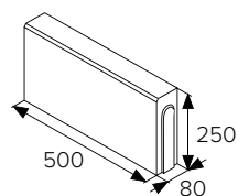
BEST LINEA I
