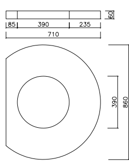
výrobní prstenec TBV-Q 390/60
