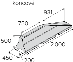
SVODIDLO MALÉ 50 koncové
