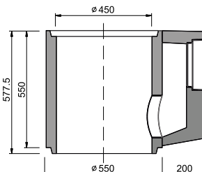
TBV-Q S/450/550 skruž se zápachovou uzávěrou DN 200 PVC
