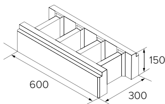
BEST MAESTRA IV (koncový poloviční prvek)
