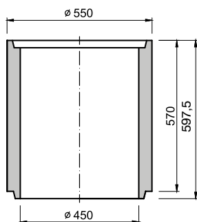
TBV-Q S/450/550 skruž se zápachovou uzávěrou DN 150 PVC
