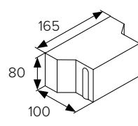
BEST BEATON rovný půlka
