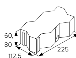
BEST BASE rovná
