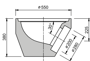
TBV-Q 1d/450/380 dno s výtokem DN 200 bez vložky
