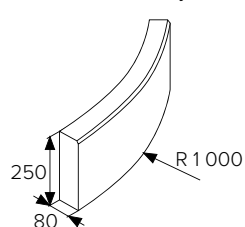
BEST LINEA R1 vnější
