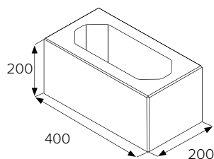
BEST MURO I
