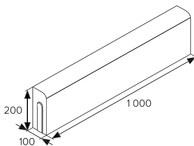
BEST SINIA II
