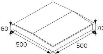
BEST ZÁKRYTOVÁ DESKA V sloupková (na sloupek 40×40 cm)
