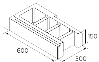
BEST MAESTRA V (rohový prvek pravý/levý)
