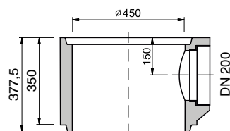
TBV-Q 3a/450/350 skruž s výtokem DN 200 PVC
