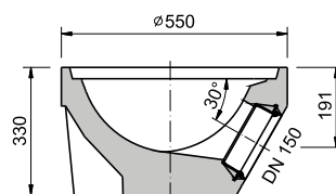
TBV-Q 1a/450/330 dno s vložkou DN 150 PVC
