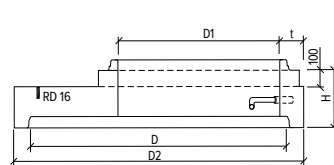
AP-MM 1500/1000×380 ZE PS
