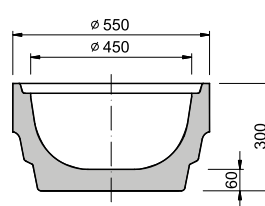
TBV-Q 2a/450/300 dno s kalovou prohlubní
