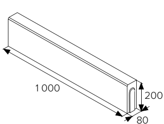
BEST LINEA III
