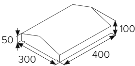
BEST ZÁKRYTOVÁ DESKA III sloupková, průběžná
