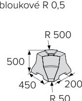
SVODIDLO MALÉ 50 obloukové R 0,5
