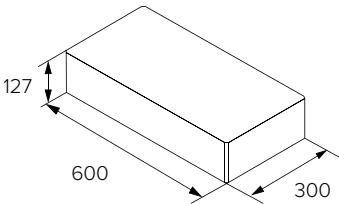
BEST ZÁKRYTOVÁ DESKA VI sloupková, průběžná (pro prvek BEST MAESTRA)
