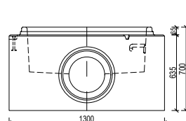
šachtové dno s výškou kynety 1-2
