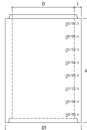
skruž SR-M 1200×2000 PS
