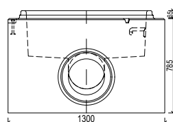
šachtové dno s výškou kynety 1-2
