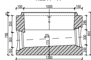
šachtové dno s náklonem ŘEZ A – A
