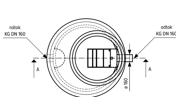
PŮDORYS
