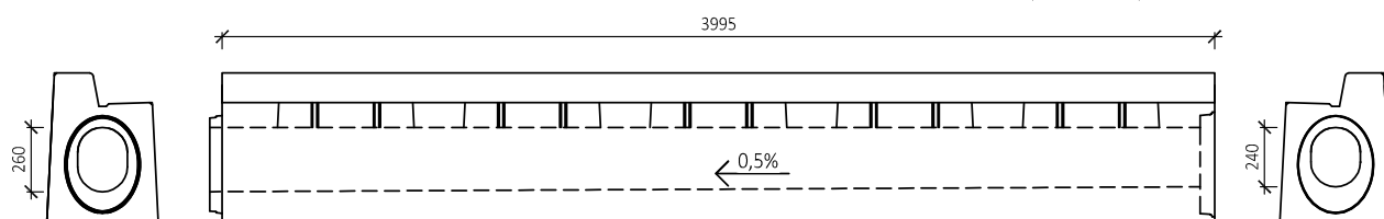
BEST TROUBA S PŘERUŠOVANÝM ŠTĚRBINOVÝM ŽLABEM, SPÁDOVÁ 20/24-26, OBRUBNÍK 12 cm (PROFIL LEVÝ)
