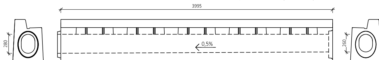
BEST TROUBA S PŘERUŠOVANÝM ŠTĚRBINOVÝM ŽLABEM, SPÁDOVÁ 20/26-28, OBRUBNÍK 12 cm (PROFIL LEVÝ)
