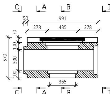
ŘEZ B-B
