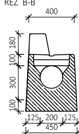
ŘEZ B-B
