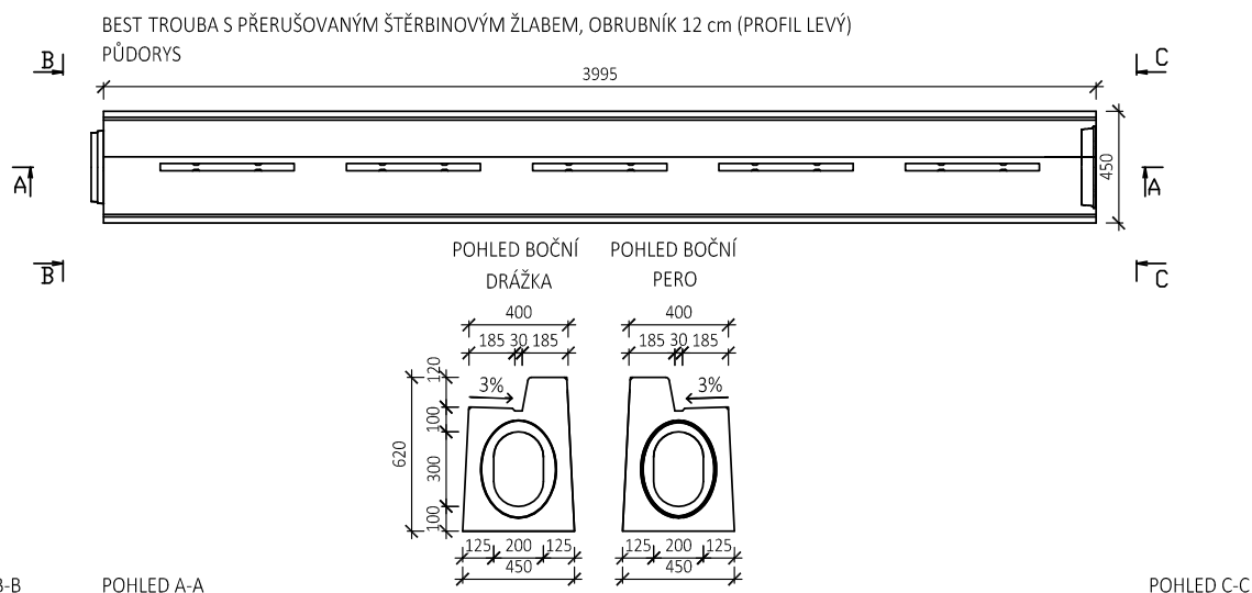
BEST TROUBA S PŘERUŠOVANÝM ŠTĚRBINOVÝM ŽLABEM, ROVNÁ, OBRUBNÍK 12 cm (PROFIL LEVÝ)
