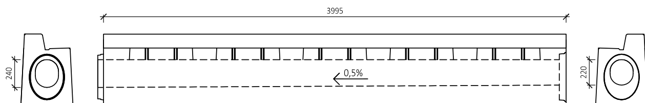
BEST TROUBA S PŘERUŠOVANÝM ŠTĚRBINOVÝM ŽLABEM, SPÁDOVÁ 20/22-24, OBRUBNÍK 12 cm (PROFIL LEVÝ)
