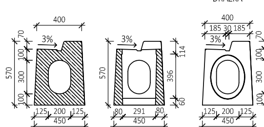
DRÁŽKA
