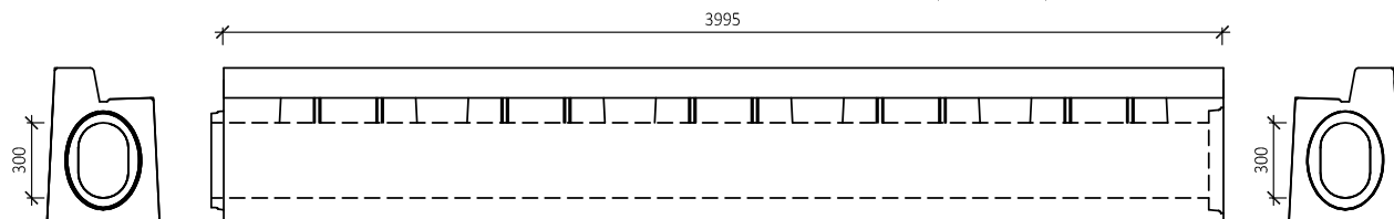
BEST TROUBA S PŘERUŠOVANÝM ŠTĚRBINOVÝM ŽLABEM, ROVNÁ, OBRUBNÍK 12 cm (PROFIL LEVÝ)
