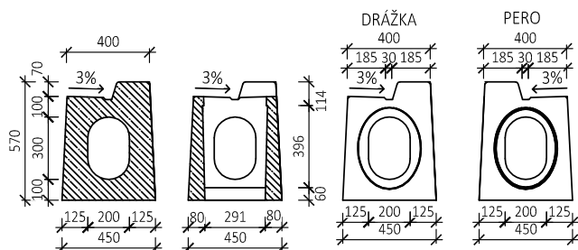
BEST VPUŠŤOVÝ KUS (DRÁŽKA-DRÁŽKA), OBRUBNÍK 7 cm (PROFIL PRAVÝ/LEVÝ)
