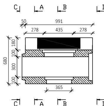
BEST VPUŠŤOVÝ KUS 20/30 (PERO-DRÁŽKA), OBRUBNÍK 18 cm (PROFIL LEVÝ)
