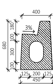
ŘEZ A-A
