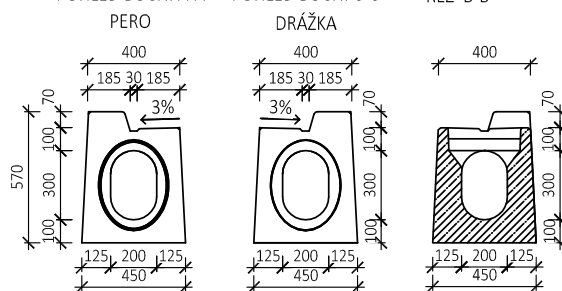
BEST VPUŠŤOVÝ KUS 20/30 (PERO-DRÁŽKA), OBRUBNÍK 7 cm (PROFIL LEVÝ)
