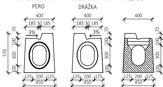
BEST VPUŠŤOVÝ KUS 20/30 (PERO-DRÁŽKA), OBRUBNÍK 7 cm (PROFIL PRAVÝ)
