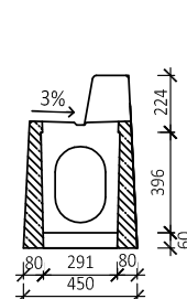
ŘEZ B-B
